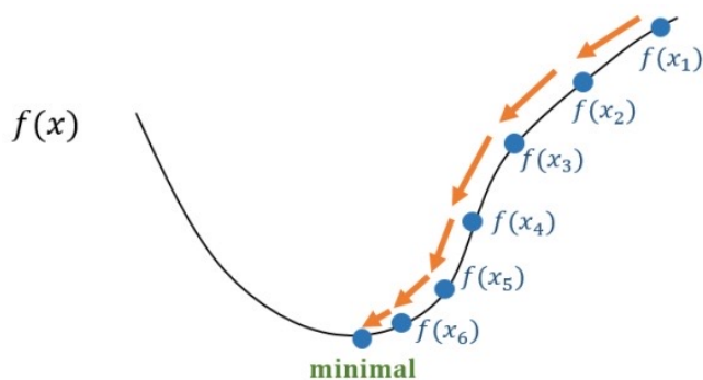
一维
