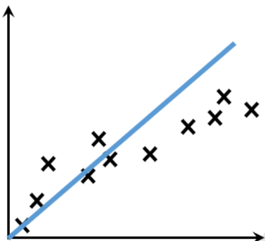
欠拟合
