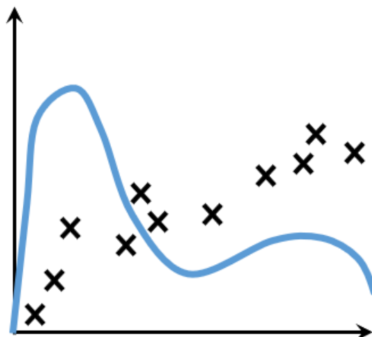
http://blog.csdn.net/miyudianzi 不收敛
